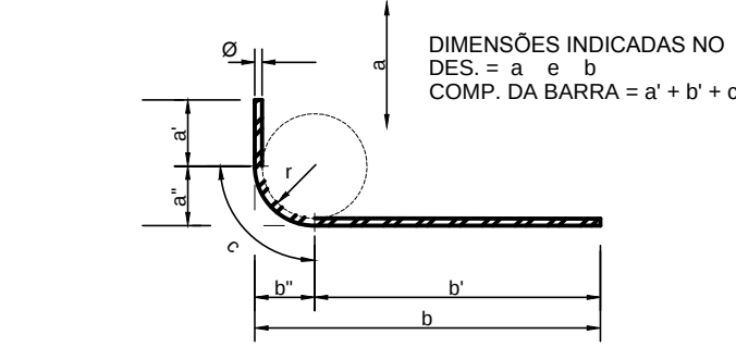
DETALHE DE DOBRA DO AÇO S/ESC.
